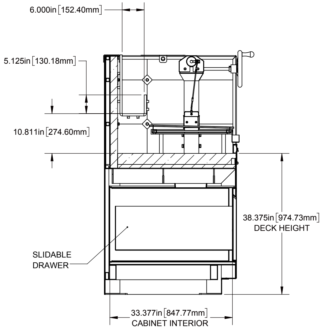
SECTION A-A SCALE 1 : 16
